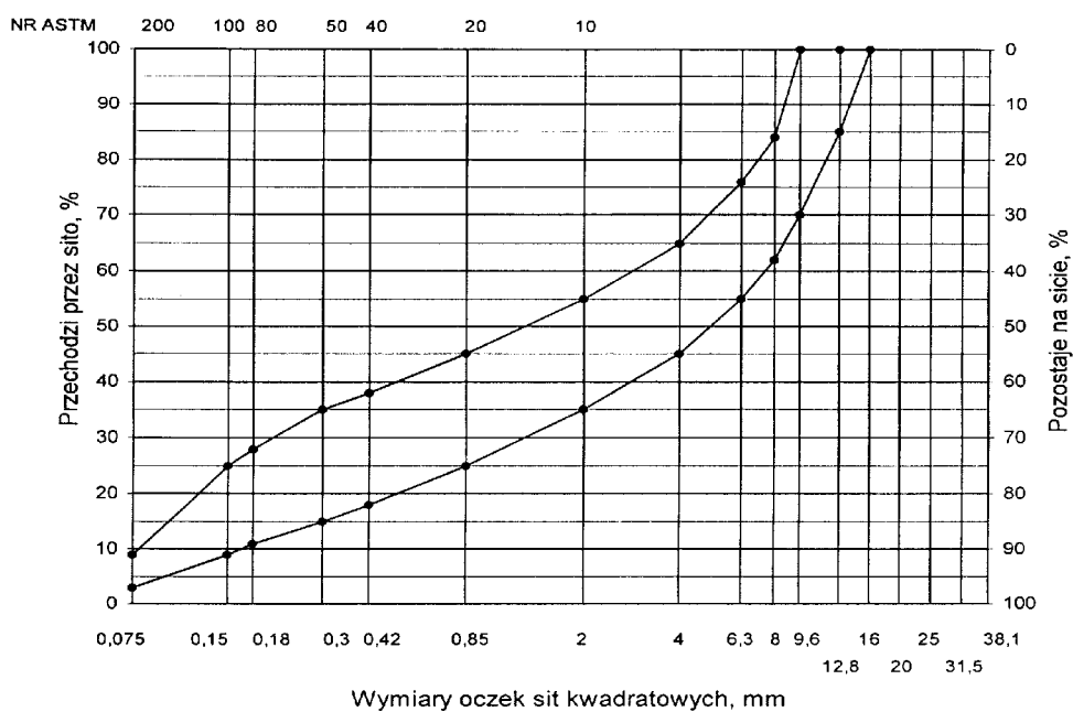
Rys. 9. Krzywe graniczne uziarnienia mieszanki mineralnej BA od 0 do 16 mm do warstwy wiążącej, wyrównawczej i wzmocniającej nawierzchni drogi o obciążeniu ruchem KR1 lub KR2
