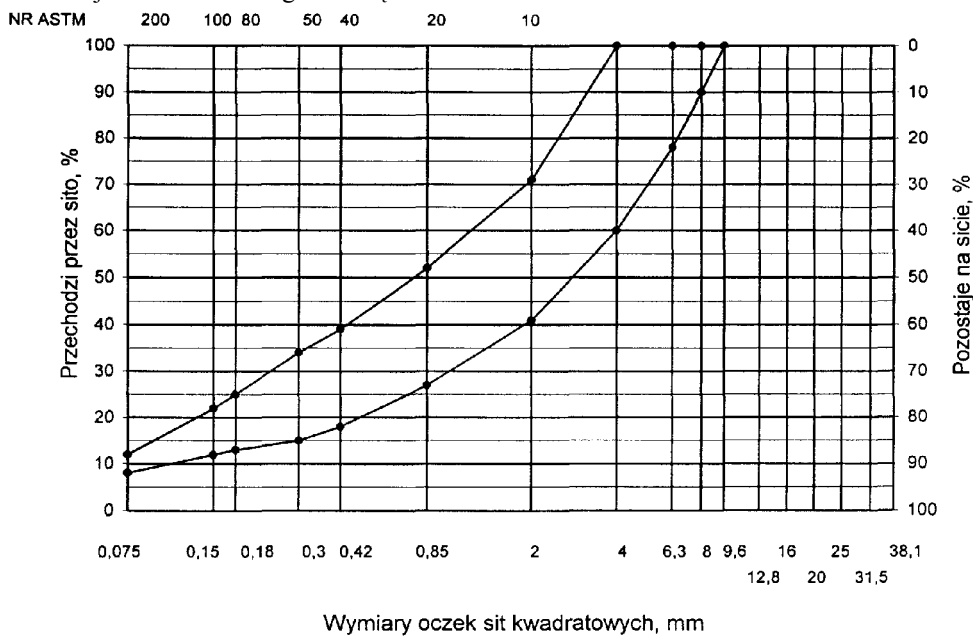
Rys. 3. Krzywe graniczne uziarnienia mieszanki mineralnej BA od 0 do 8mm, od 0 do 6,3 mm do warstwy ścieralnej nawierzchni drogi o obciążeniu ruchem
